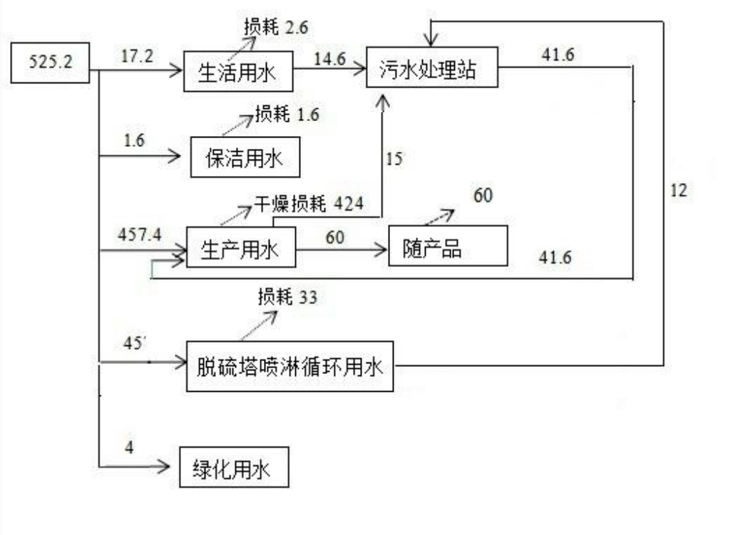
图1 给排水平衡图 (单位: t/d )
